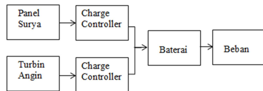
Gambar 3.1. Skema sistem pada alat
