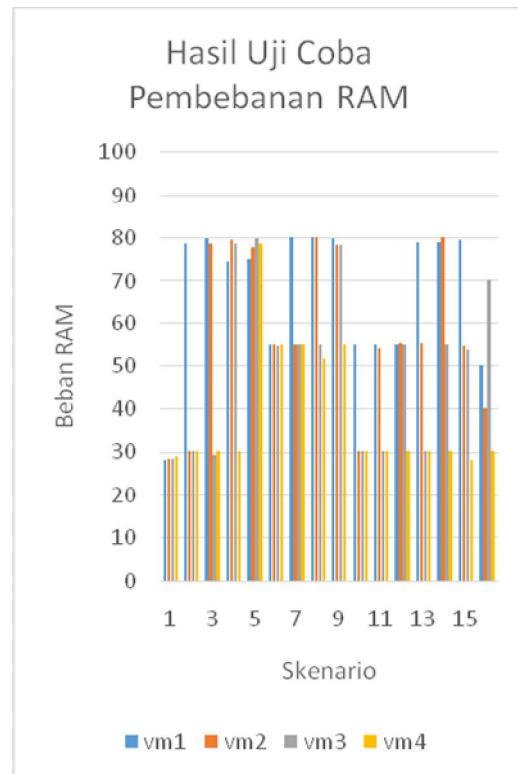
Gambar 5. Hasil Uji Coba Pembebanan RAM
