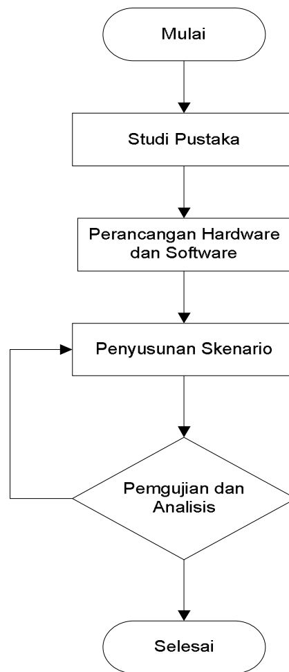
Gambar 2. Tahapan Penelitian
