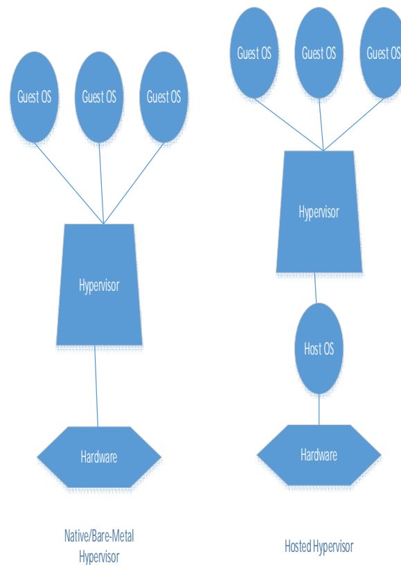
Gambar 1. Jenis-Jenis Hypervisor
