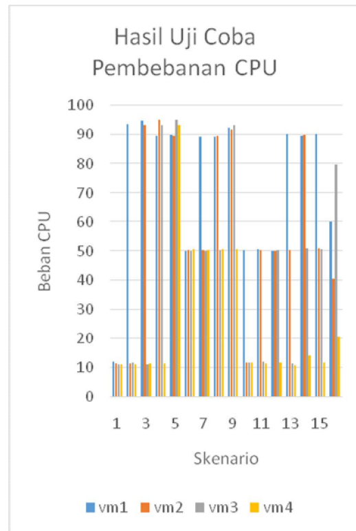
Gambar 4. Hasil Uji Coba Pembebanan CPU
