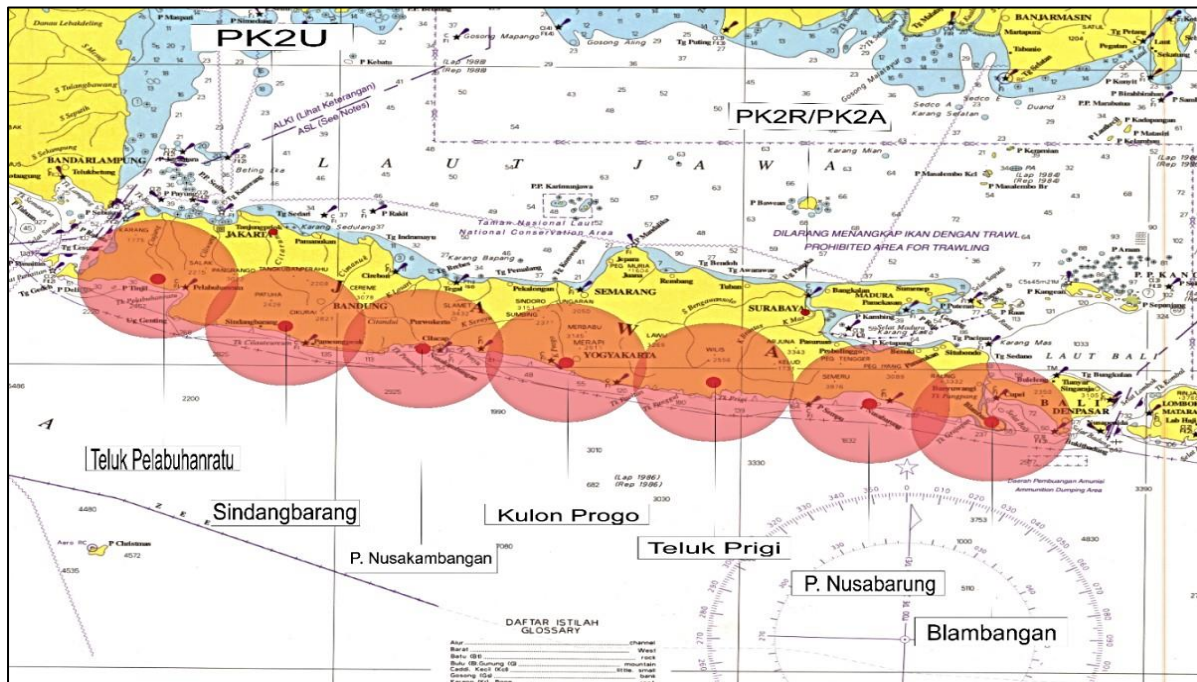
Gambar 3. Konsep pemasangan radar SJCSS
