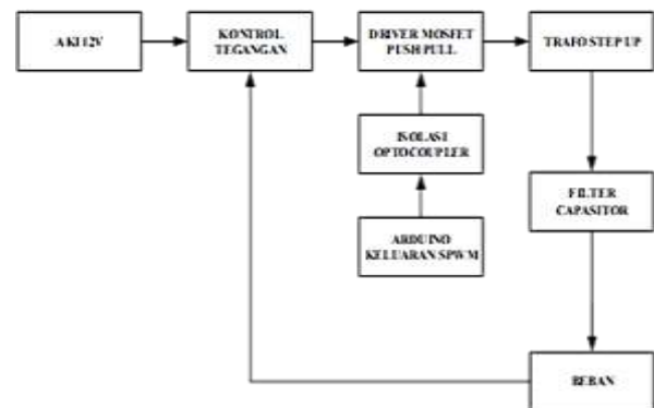
Gambar 2. Blok Diagram Perangkat Keras dari Inverter SPWM
