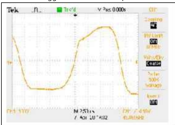
Gambar 17. Hasil Pengamatan Satu Periode Keluaran Inverter SPWM Setelah Menggunakan Beban
