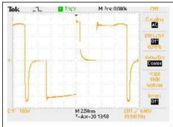
Gambar 9. Hasil Pengamatan Keluaran Inverter Square Wave Tanpa Menggunakan Beban
