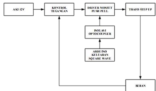
Gambar 3. Blok Diagram Perangkat Keras dari Inverter Square Wave
