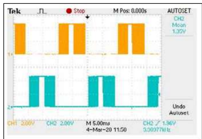
Gambar 7. Hasil Pengamatan Pembangkit SPWM Menggunakan Osiloskop
