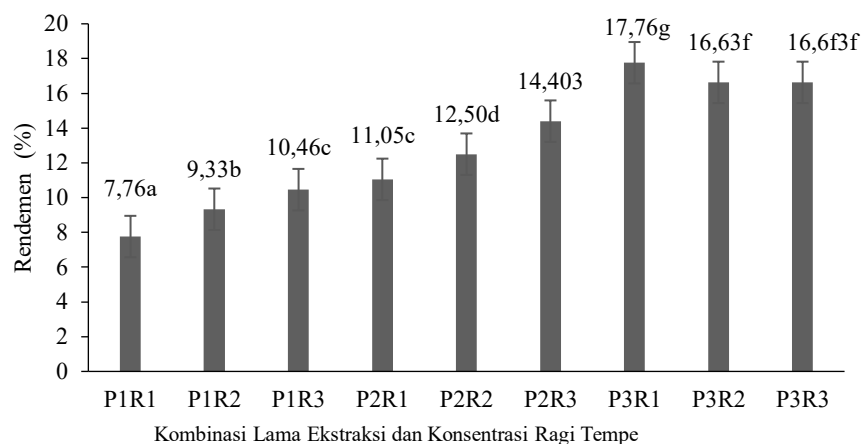
Gambar 3 Kombinasi perlakuan lama ekstraksi dan konsentrasi ragi tempe terhadap rendemen minyak kelapa
